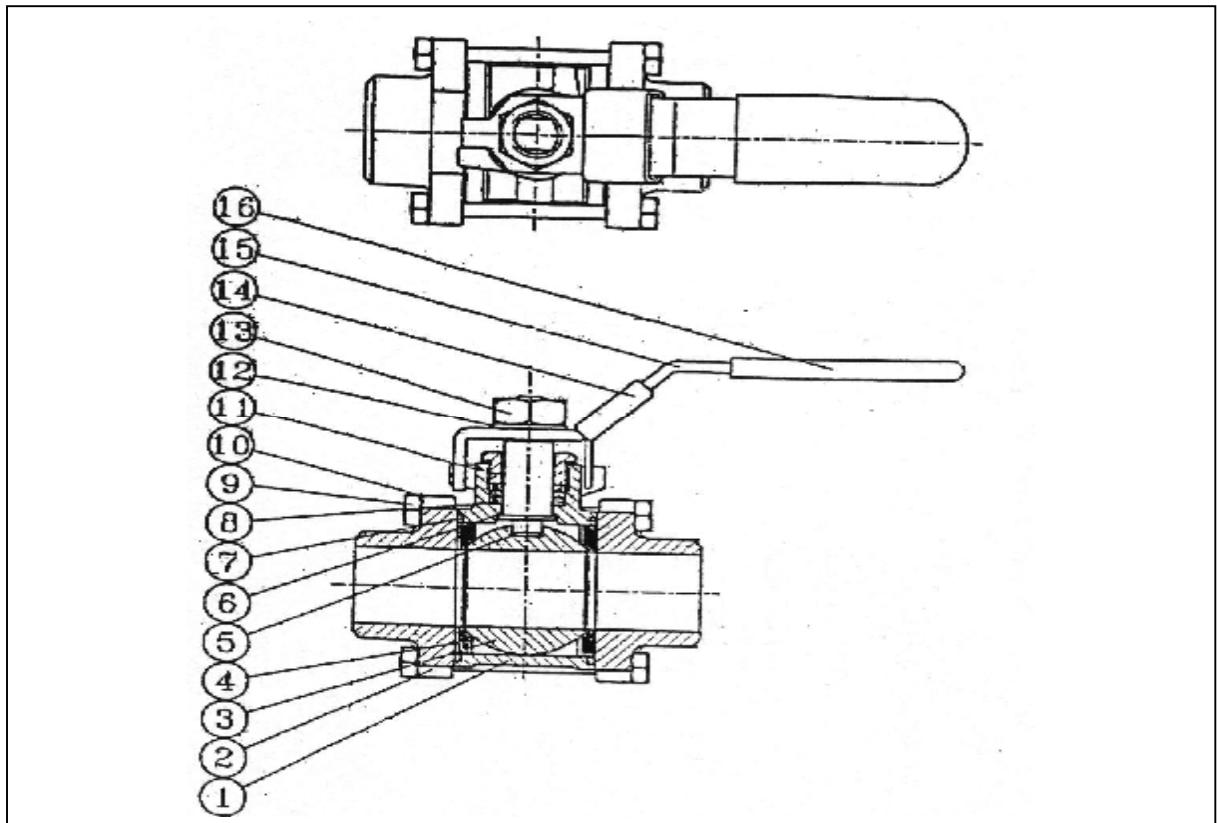
Рис. 24. Устройство шаровых кранов тип Х3777 (В,С), Х3888(В,С), Х3777V.
