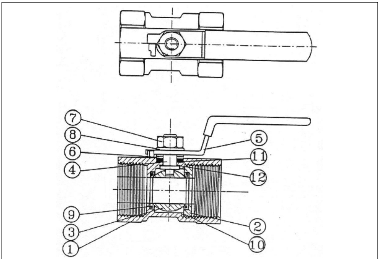
Рис. 4. Устройство шарового крана тип X1666.
