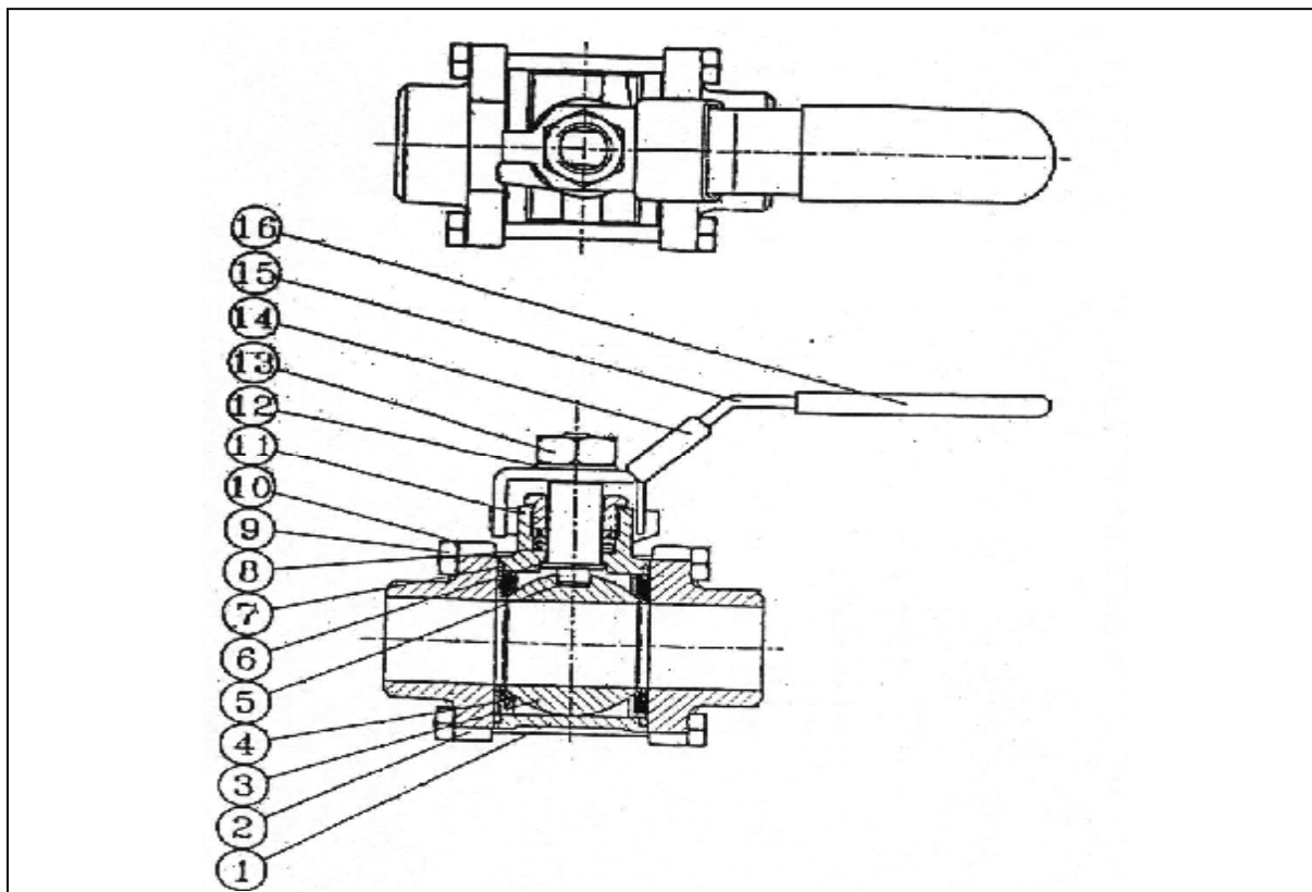
Рис. 18. Устройство шаровых кранов тип X3444 (B,S), X3555(B,S)
