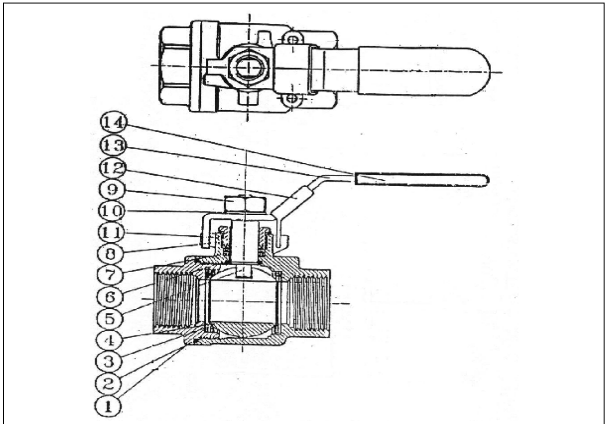
Рис. 8. Устройство шарового крана тип X2777.
