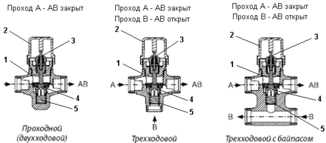
Рис.4. Устройство клапанов.
