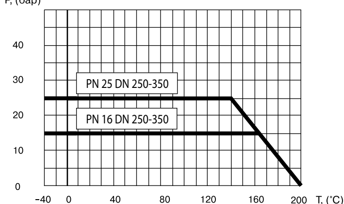
График «Температура-Давление»
