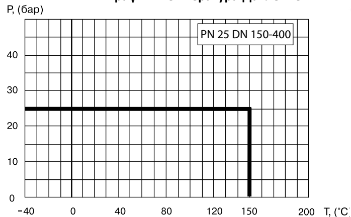
График «Температура-Давление»
