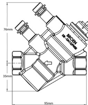
Рис. 37 Установочные размеры клапана БРОЕН Dynamic
