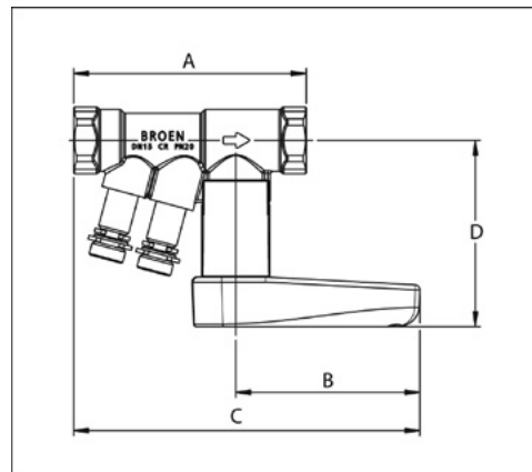
Рис. 57 БРОЕН Venturi
