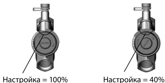
Рис. 39 Грубая настройка клапана БРОЕН Dynamic на расчетный расход (без расходомера)
