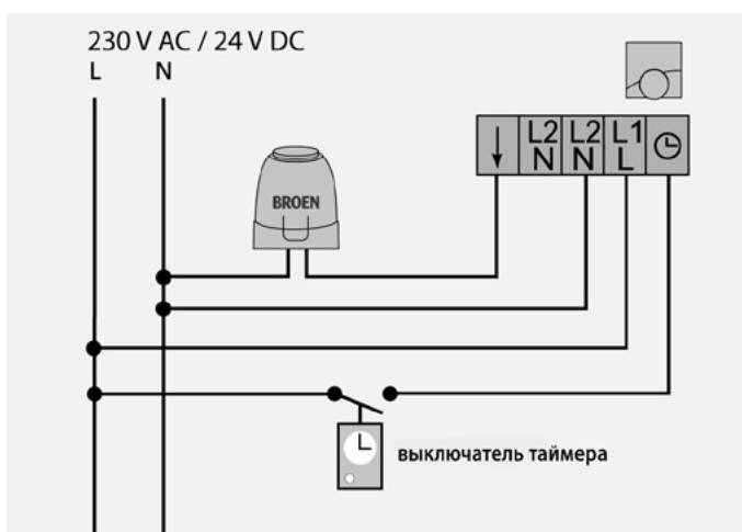
Рис. 55 Схема подключения привода
