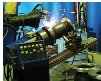
Приварка фланцев
