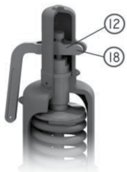
подъемник
