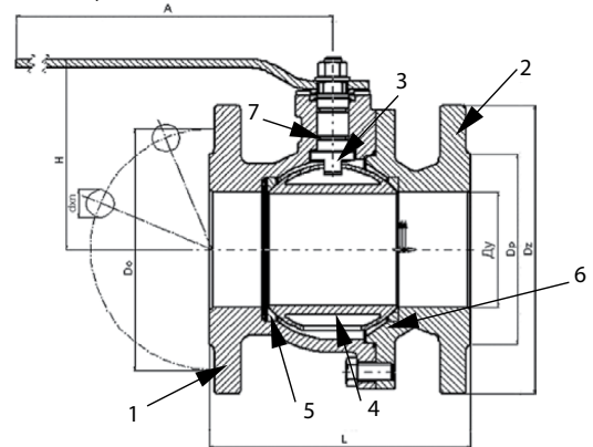
DN 015, DN 080-150
